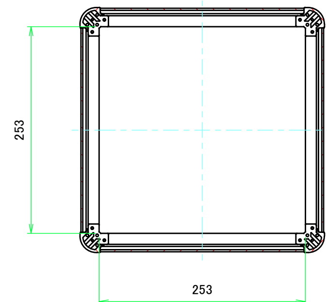
C-C ( 1 : 4.5 )
